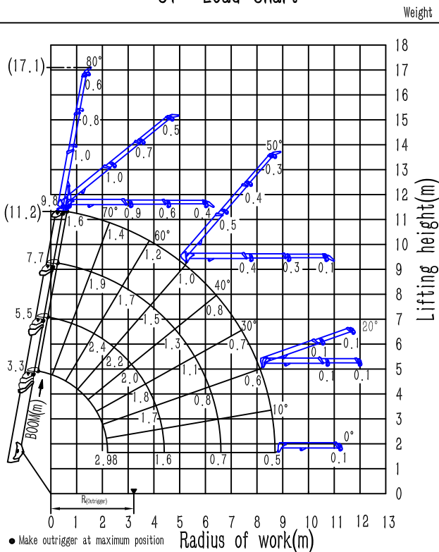
S7—Load Chart
